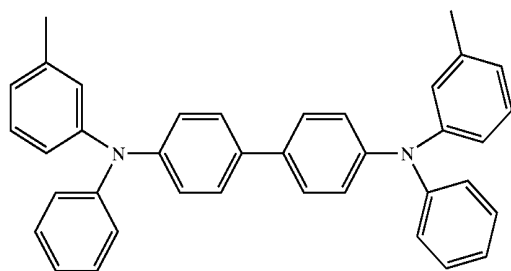
TPD
