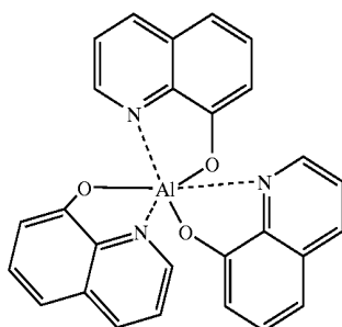
AlQ3
