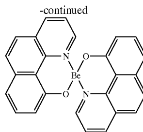
Bebq2
